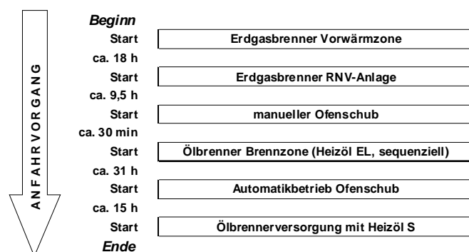
Abb. 14: Ablaufschema des Anfahrvorgangs am Tunnelofen im Ziegelwerk
