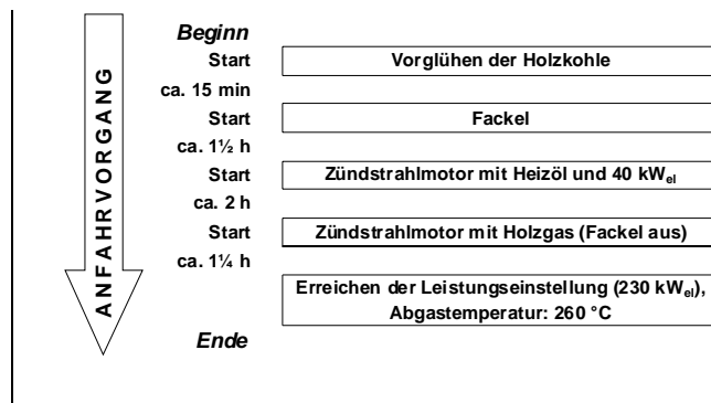
Abb. 20b: Ablaufschema des Anfahrvorgangs an der Holzgasverstromungsanlage
