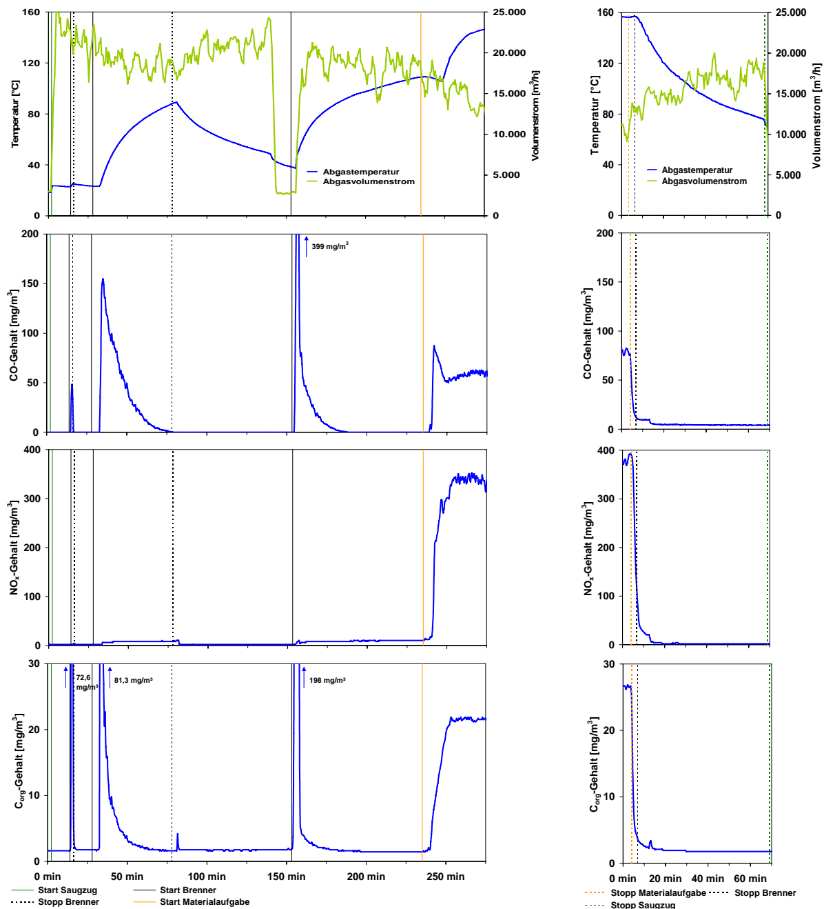
Abb. 7: Verläufe von Abgastemperatur und -volumenstrom sowie der Abgasgehalte an Kohlenstoffmonoxid, Stickstoffoxiden und organischem Gesamtkohlenstoff während des An- (links) und Abfahrens (rechts) der Glasschäumenlage
