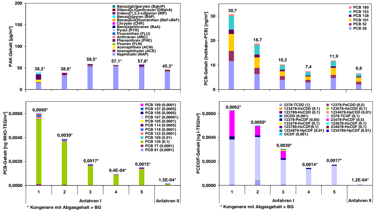
Abb. 12: Abgasgehalte an PAK, Indikator-PCB, coplanaren PCB (WHO) und PCDD/F während der Anfahrvorgänge I (Probennahmephase 1 bis 5) und II des Zementwerks; BG: Bestimmungsgrenze
