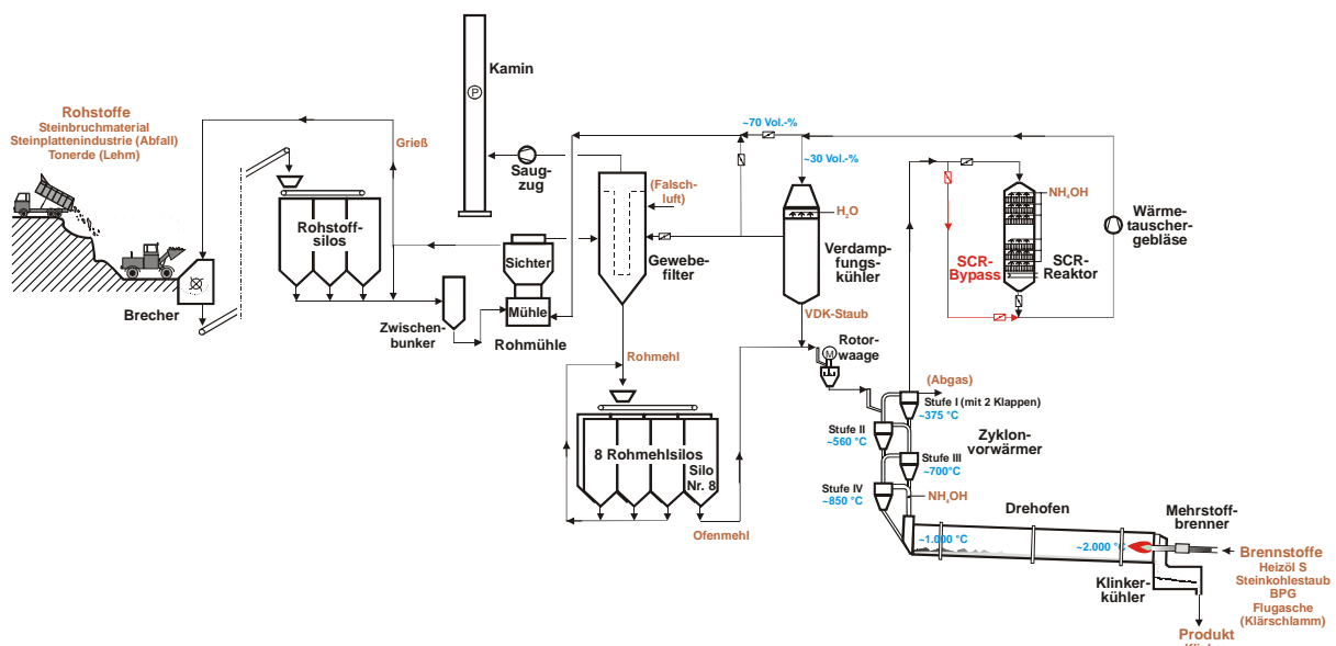
Abb. 9: Zementwerk – Verfahrensschema mit eingerichteter Probenahmestelle (P) im Reingas (am Kamin)
