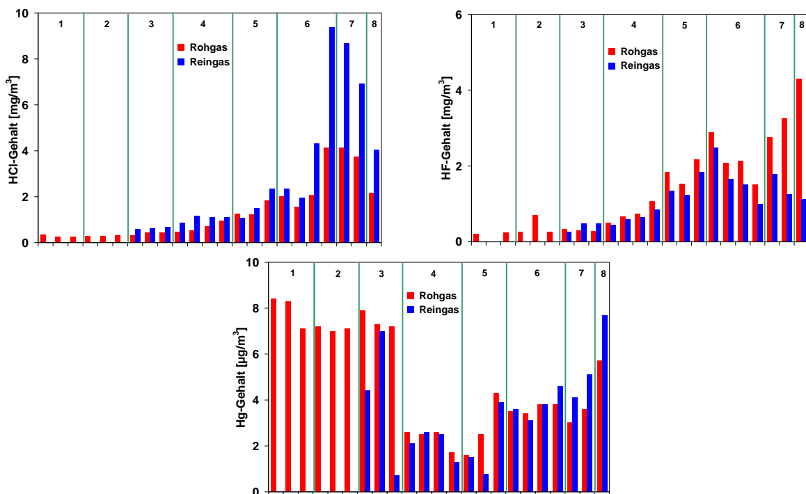
Abb. 16: Roh- und Reingasgehalte (Halbstundenmittelwerte) an Chlor-, Fluorwasserstoff und Quecksilber in den Probennahmephase 1 bis 8 während des Anfahrens des Tunnelofens
