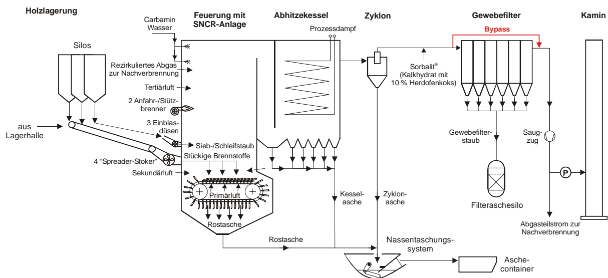
Abb. 23: Holzheizkraftwerk – Verfahrensschema mit eingerichteter Probenahmestelle (P) im Reingas (vor Kamin)
