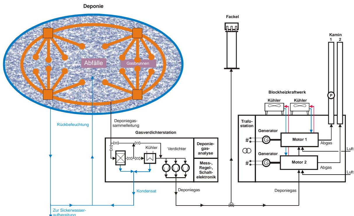
Abb. 18: Deponiegasverstromungsanlage – Verfahrensschema mit eingerichteter Probenahmestelle (P) im Reingas (am Kamin 1)
