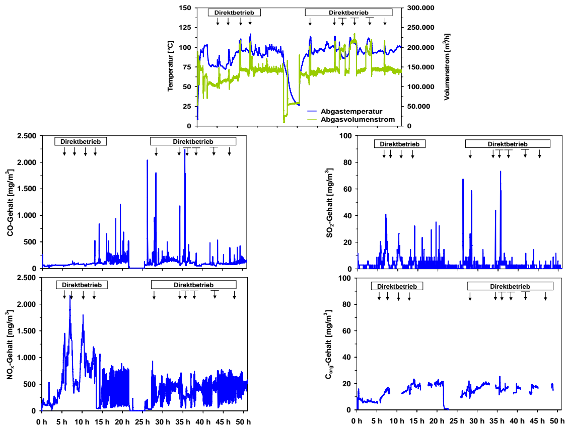
Abb. 11: Verläufe von Abgastemperatur und -volumenstrom sowie der Abgasgehalte an Kohlenstoffmonoxid, Schwefeldioxid, Stickstoffoxiden und organischem Gesamtkohlenstoff im Reingas während des Anfahrens des Zementwerks
