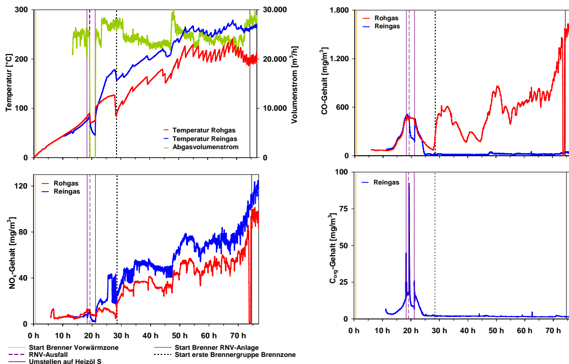
Abb. 15: Verläufe von Abgastemperatur und -volumenstrom sowie der Abgasgehalte an Kohlenstoffmonoxid, Stickstoffoxiden und organischem Gesamtkohlenstoff im Roh- und Reingas während des Anfahrens des Tunnelofens
