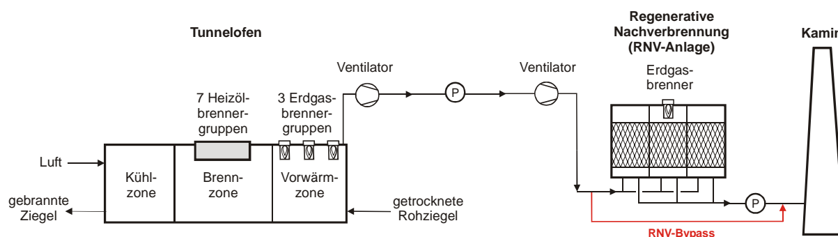
Abb. 13: Ziegelwerk – Verfahrensschema mit den eingerichteten Probenahmestellen (P) im Roh- (nach Tunnelofen) und Reingas (vor Kamin)
